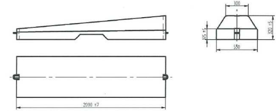
Bariera A typ BPPS-1 – najazdowa – stała skrajna dwustronna L=2 m
