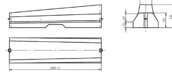
Bariera B typ BPPS-1 – najazdowa – stała skrajna dwustronna L=2 m
